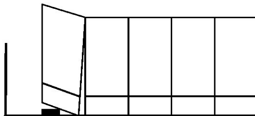
Схема размещения пакетов в кузове грузового транспортного средства с применением бруска
